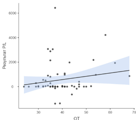
Рис. 3. Діаграма розсіювання
